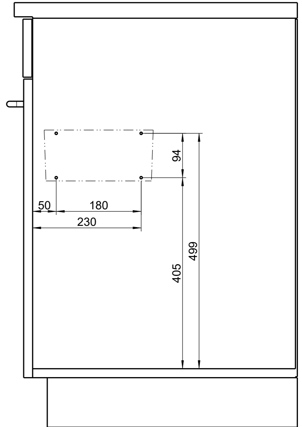
Bohrbilder: Front / Kastenboden / Seitenwand L+R
